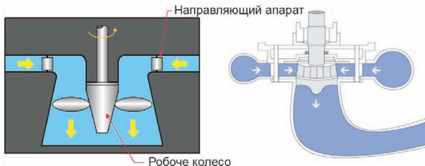
Пропелерна турбіна 5
