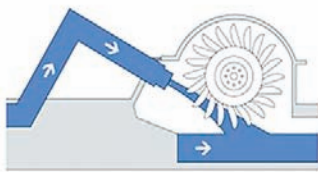
Ковшова турбіна 2
