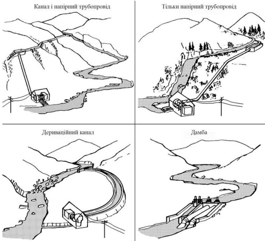
Малюнок 3-8: Найбільш розповсюджені схеми малих гідроелектростанцій
