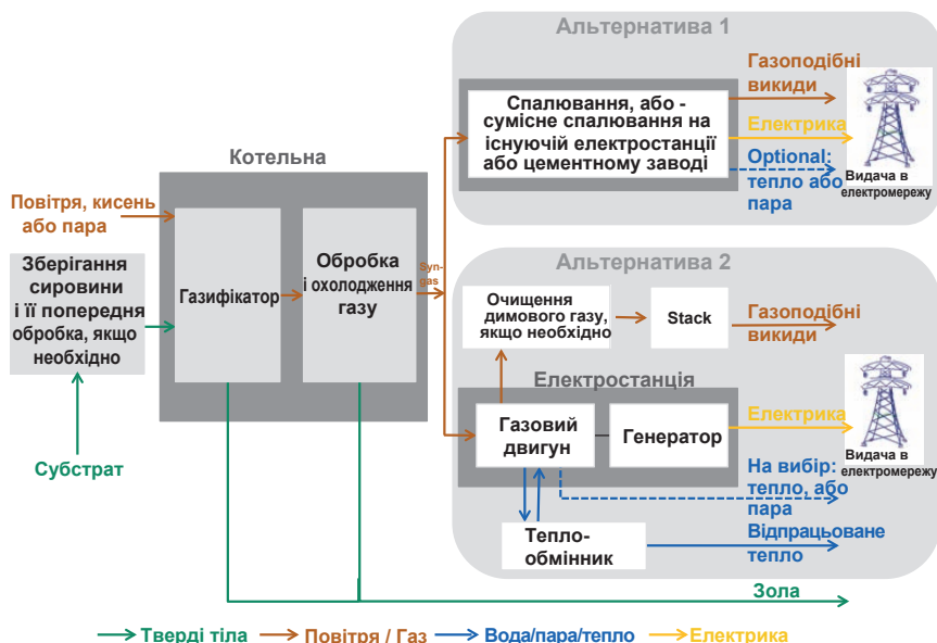
Малюнок 3-19: Блок-схема установки для перетворення біомаси в енергію, основаної на процесі газифікації
