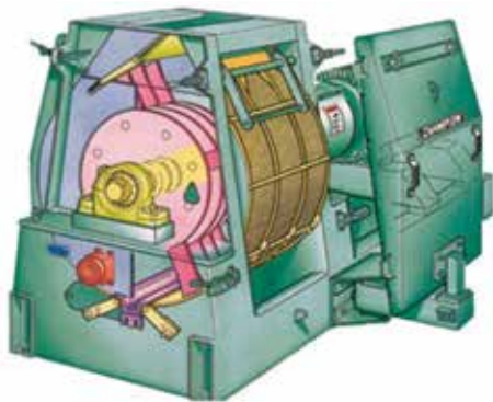
б) молоткова дробарка тину Champion (СРМ) 12
