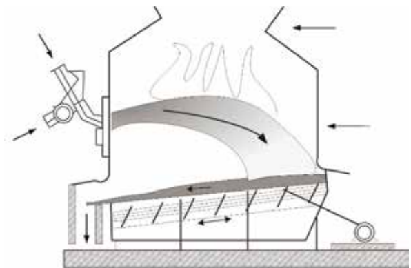
Рис. 4.8. Вібраційна решітка з пневмо-закидачем палива
