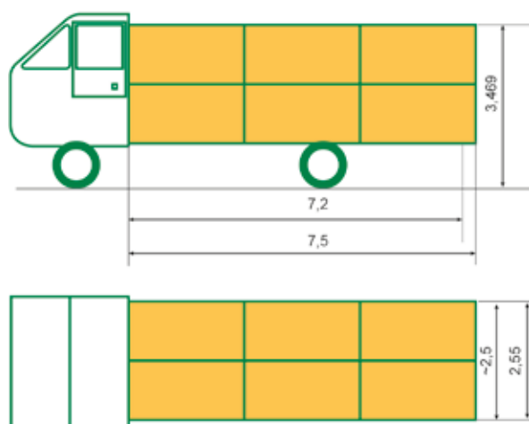
Рис. 3.22. Схема розміщення 12-ти тюків соломи на вантажівці
