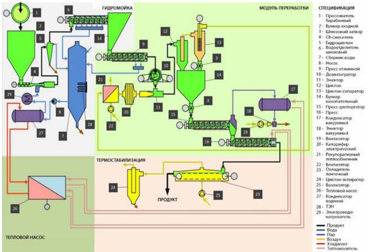
Рис. 4.29. Схема влажного пресования на примере работы компании BM Engineering
