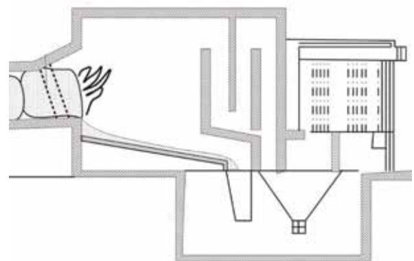
Рис. 4.9. Сигарне спалювання туків соломи з допалюванням на вібраційній решітці
