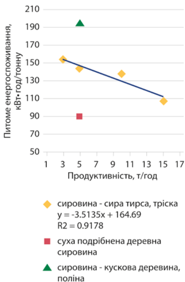
Рис. 3.45. Питоме електроенергоспоживання залежно від масштабу виробництва 41, 42
