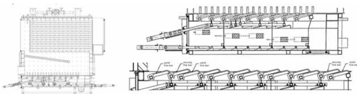
Рис. 5.20. Конструкція рухомих ґрат котла GRANPAL MEGA
