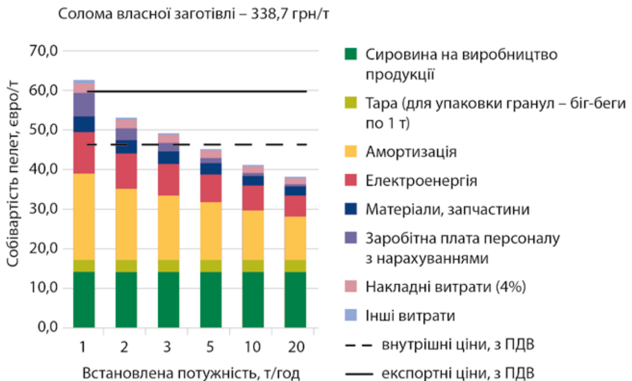
Рис. 5.5. Розрахункова собівартість виробництва пелет із соломи
