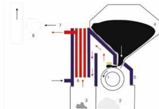
Рис. 4.12. Схема котла Carborobot
