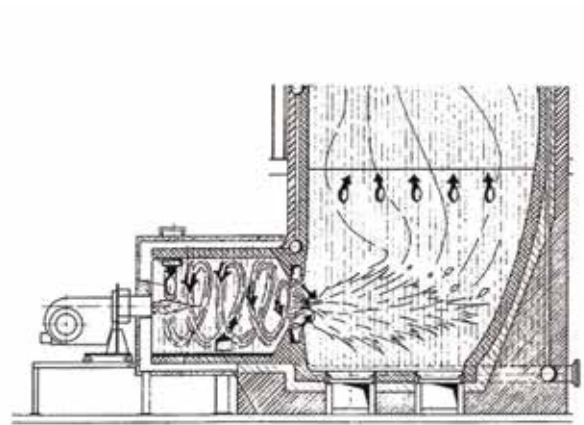
Рис. 4.21. Використання попередньої газифікації БМ у поєднанні з водотрубним котлом
