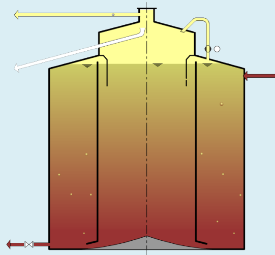
Гідравлічний реактор
